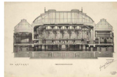
Giergl első metszeti terve, mely változott
